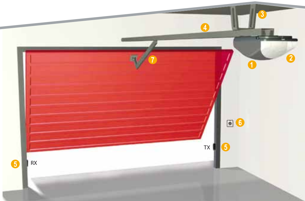
Motor with control board and internal 433,92 MHz radio receiver Motoriduttore con centrale di gestione e ricevitore 433,92 MHz incorporati
